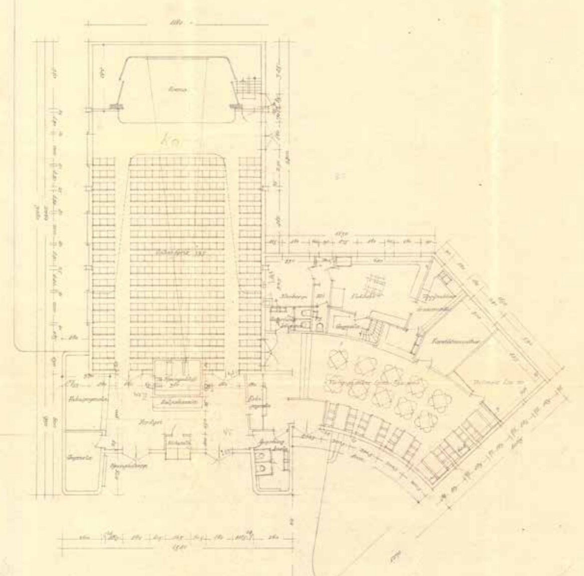
Grunnteikning af Selfossbíó og veitingasölu Hótel Selfoss, ótímasett. Teiknað af Gunnlaugi Halldórssyni arkitekt, yfirmiður var Guðmundur Eiríksson. Húsið var í alla staði hið glæsilegasta með sal fyrir 335 gesti og stóru sviði. Veitingasalur tók 80 manns í sæti. Þarna komu Selfyssingar saman og skemmtu sér, haldnir voru dansleikir, fundir, leiksýningar og námskeið. Sannkallað menningarhús. Teikningin kemur úr safni Guðmundar Helga Eiríkssonar (1899-1984), Merkgarði. 2021/106 Guðmundur Eiríksson, Merkgarði A/1 - 3.
