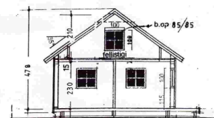
SNÍÐ A-A
