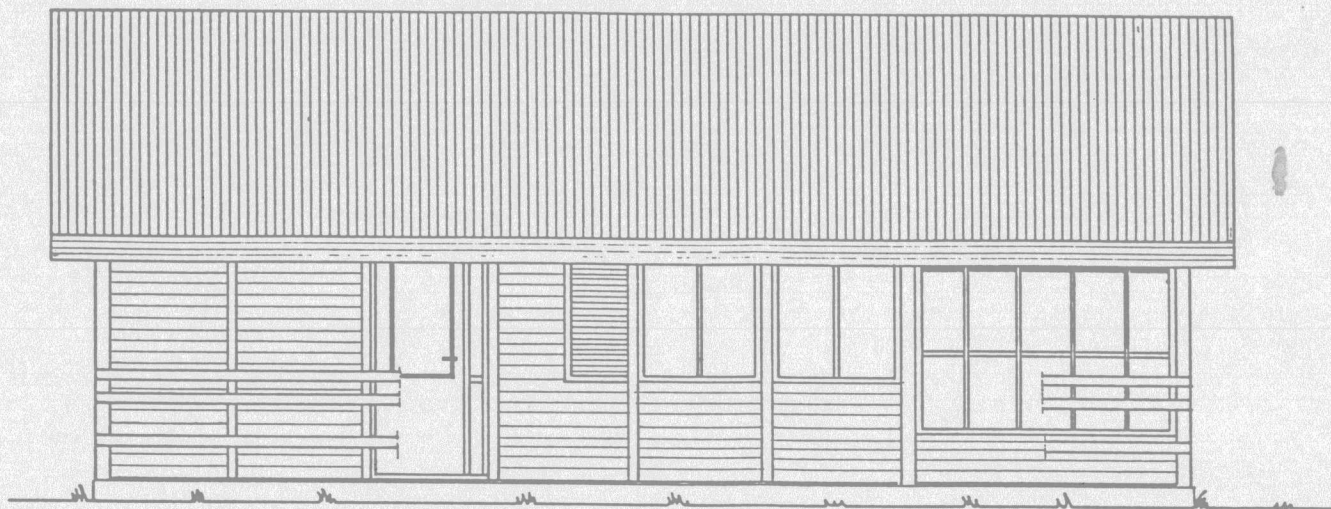
VESTLÆG HLIÐ 1:50
