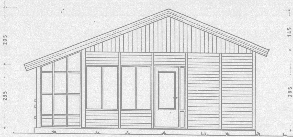
SUÐLÆG HLID 1:50
