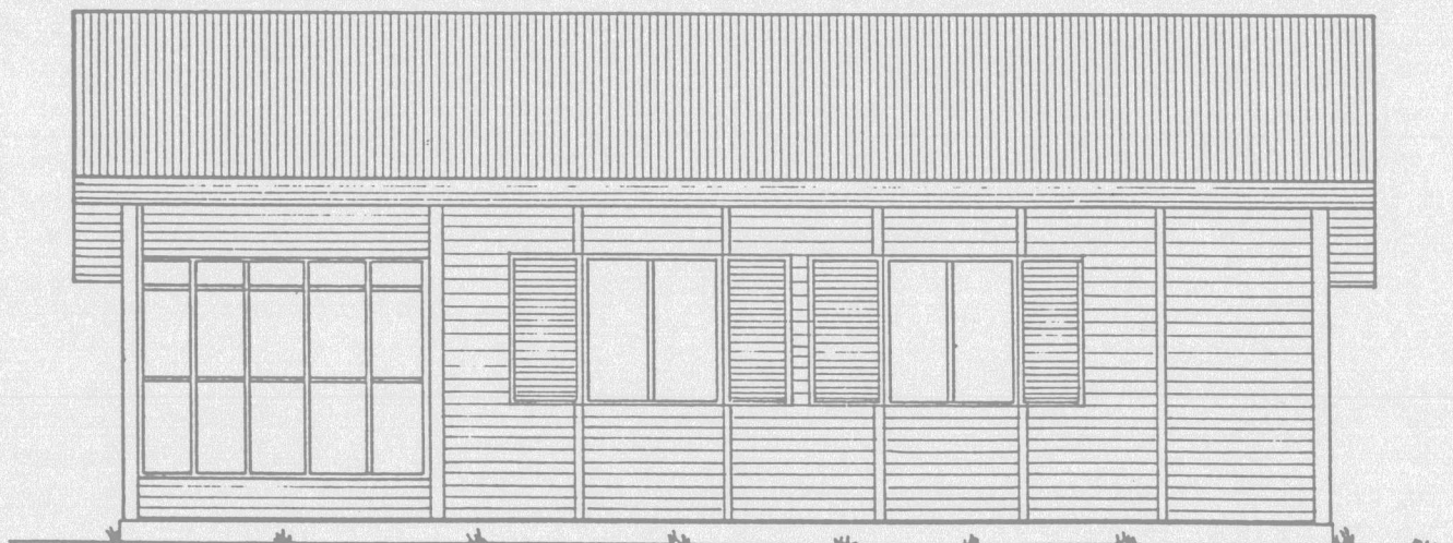
AUSTRÆG HLIÐ 1:50
