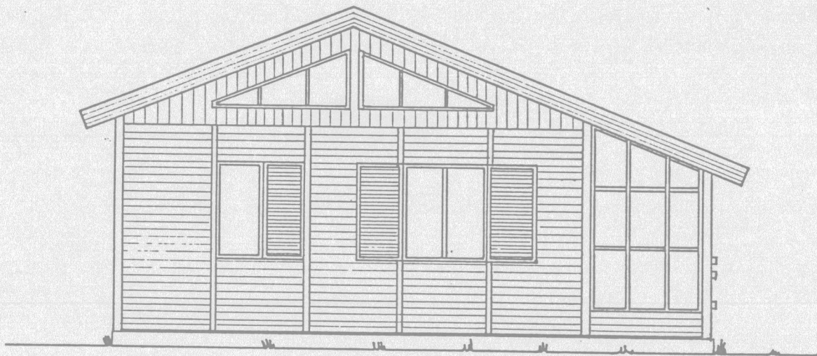
NORÐLÆG HLID 1:50
