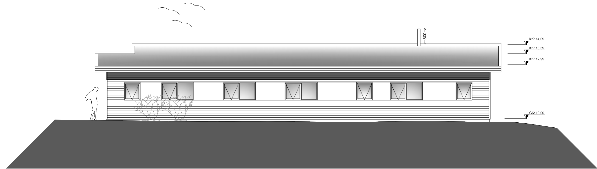
Útlit - Norður
