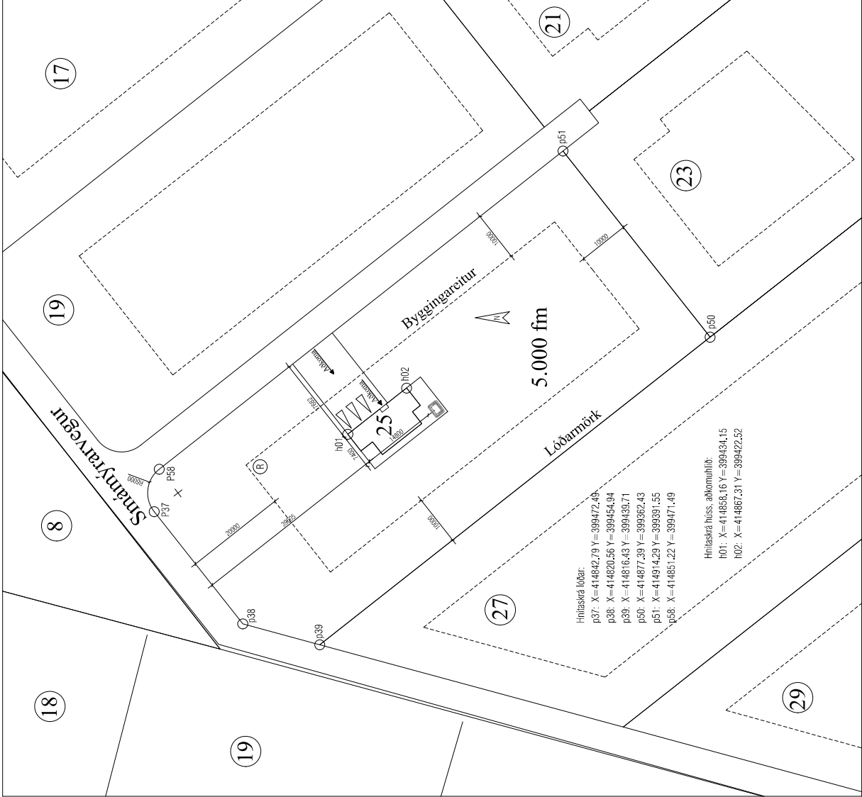
Áfstöðumynd 1:500
